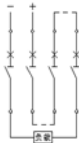
4P 外形 G1 型
