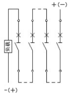
4P 外形 4 极串 3
