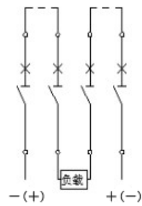
4P 外形 4 极串 1
