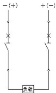
3P 外形 2 极串
